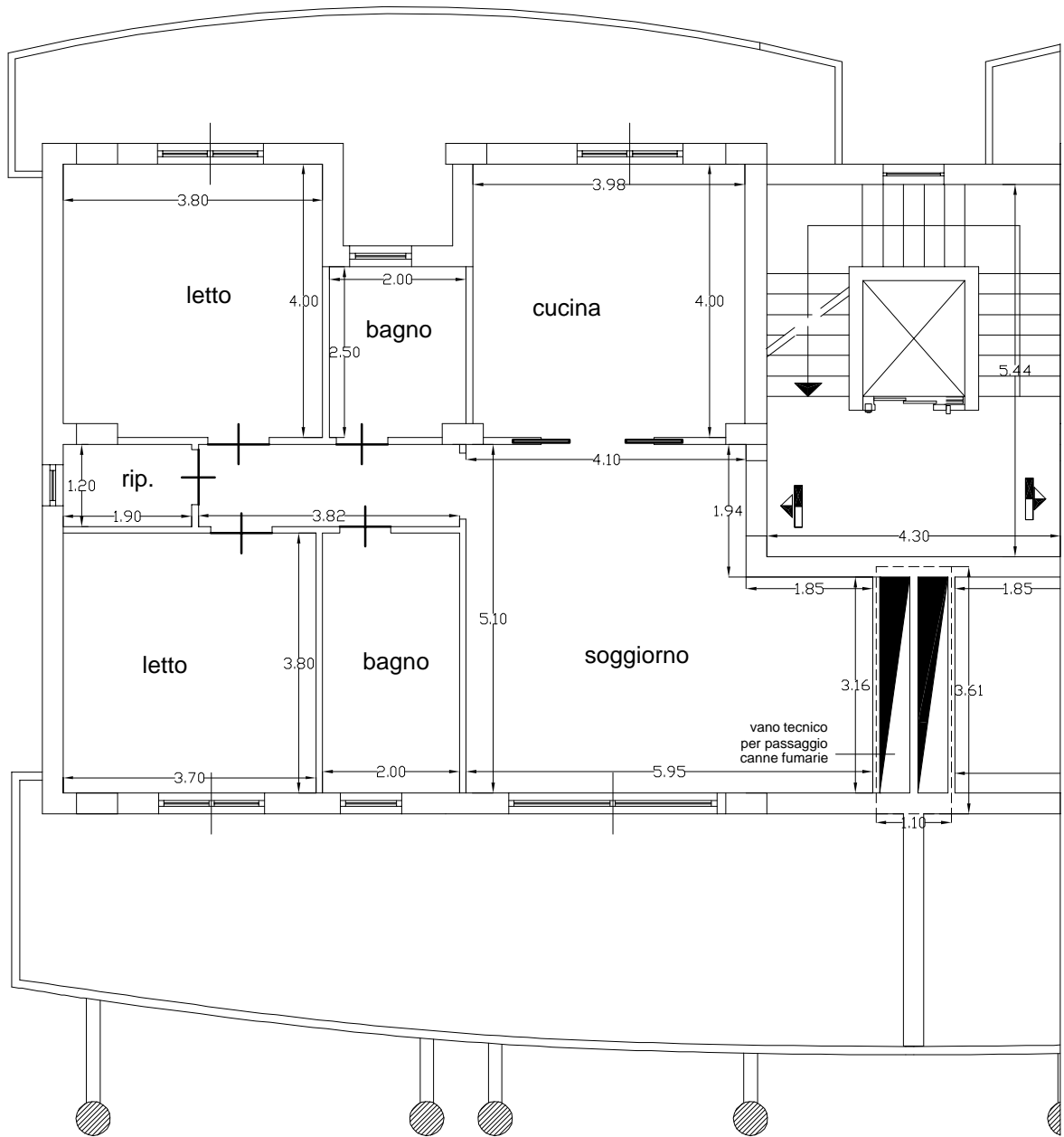
PIANTA PIANO 1° (quota + 4,15 mt.)
