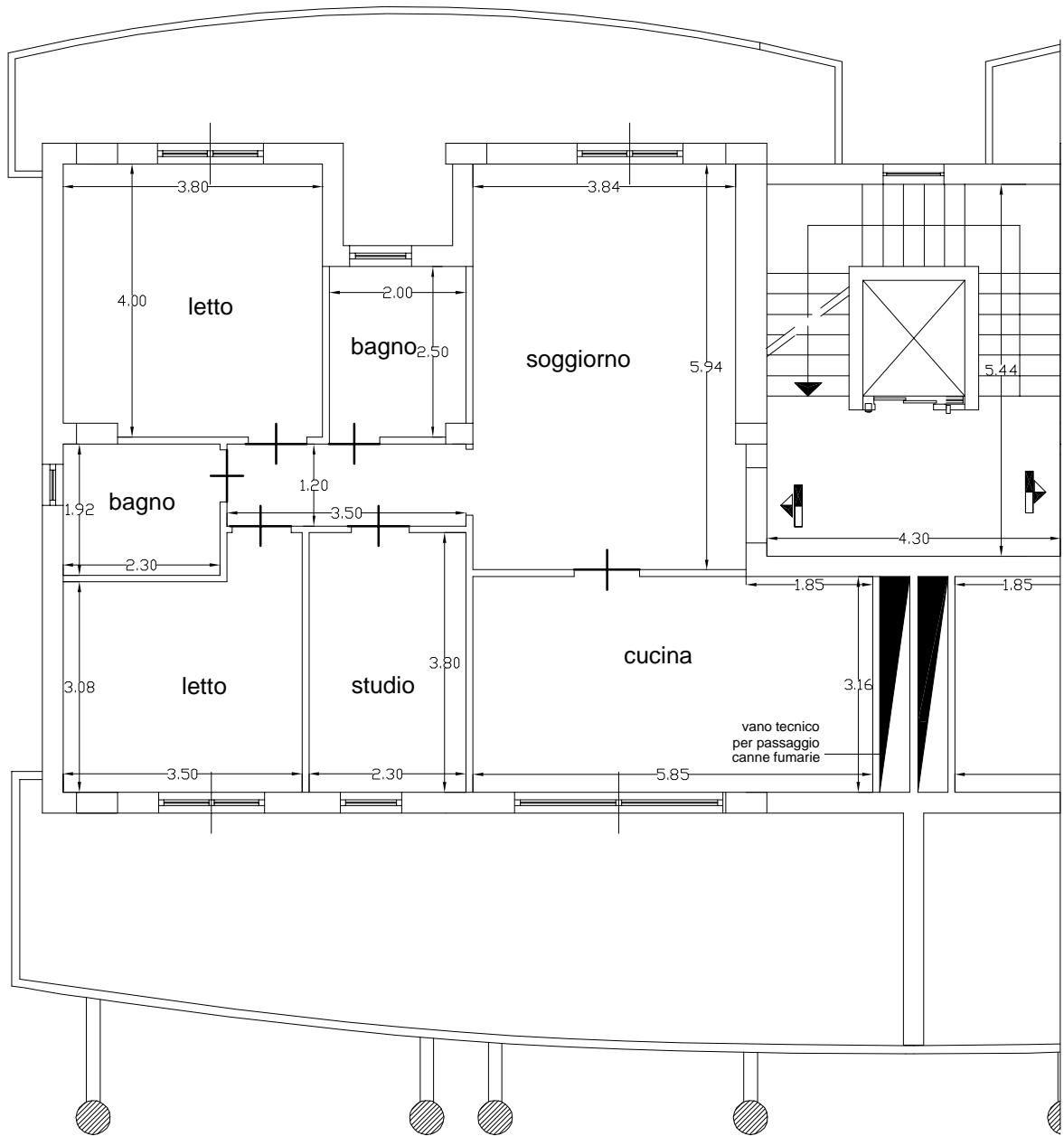
PIANTA PIANO 2° (quota +7,35 mt.)
