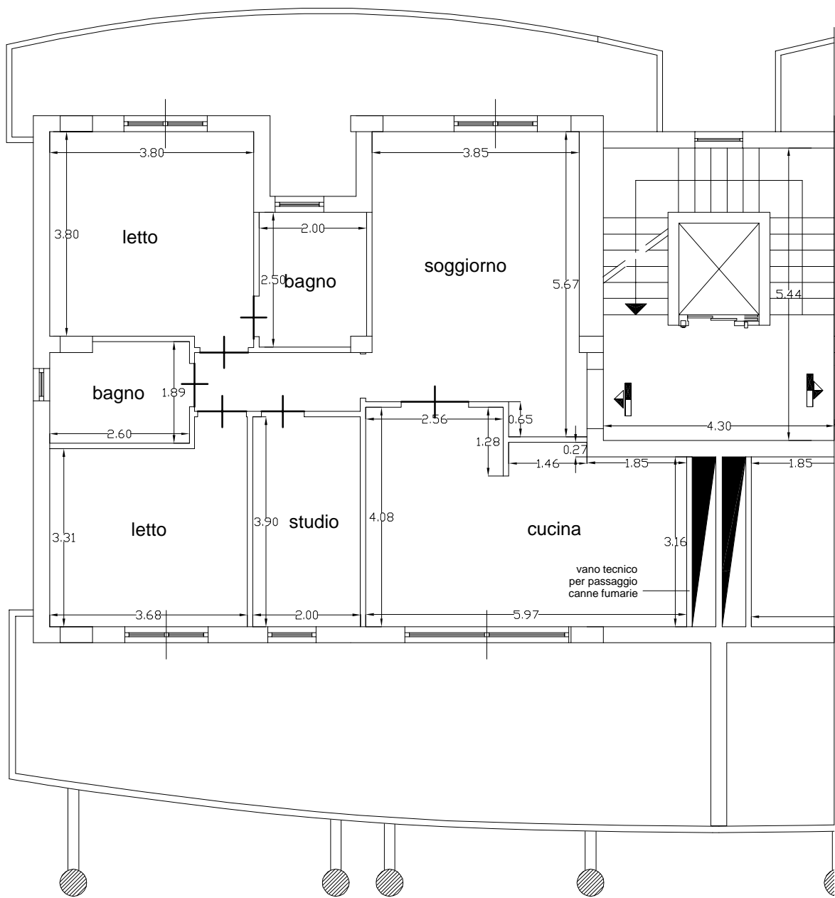
PIANTA PIANO 3° (quota +10,55 mt.)
